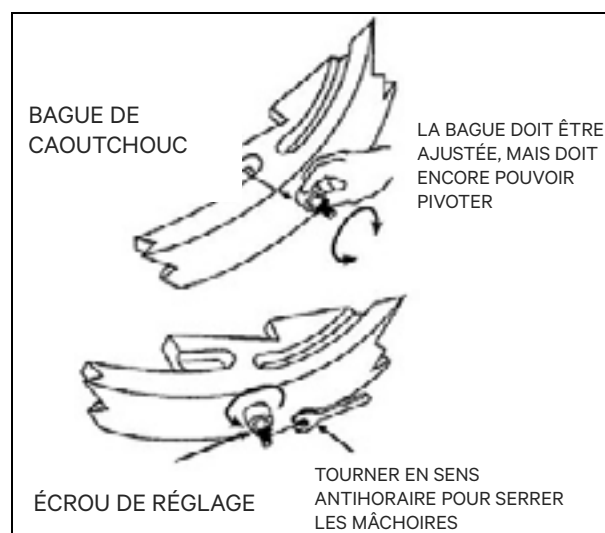
Figure 50 – Réglage – Mécanisme de verrouillage
