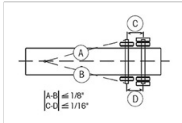
Figure 29 – Schéma de mesure
