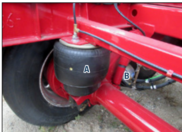
Figure 31 – Coussins pneumatiques (type)
